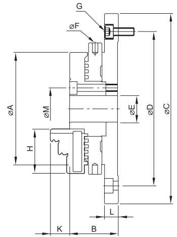
尺寸圖 / DIMENSIONS
